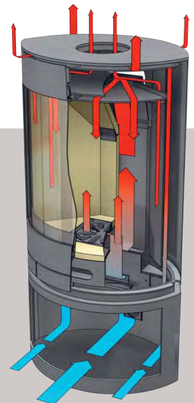
Circolazione dell'aria all'interno della stufa camino
